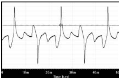
Obr. 13. Průběh primárního proudu popisovaného transformátoru 20 VA při zatížení zdroje ss proudem 100 mA. Naše zapojení z obr. 2 – 40 mA, klíčový proud TDA2009 60 mA.
