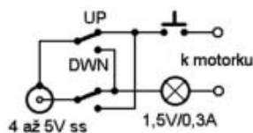
Obr. 6. Jednoduché zapojení obvodu napájení přeladovacího motorku.
