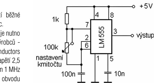
Obr. 3. Obvod pro řízení LED diody napětím s proměnnou střídou
