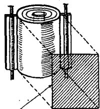
F_{cm^2} = Na w
