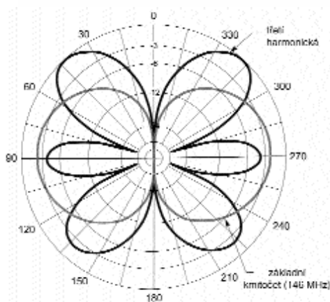
Obr. 2. Porovnávací vyzářovací diagramy dvou antén v horizontální rovině. Modelováno programem EZNEC.
