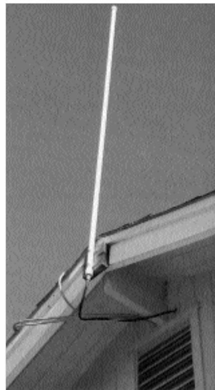
Obr. 3. Hotová anténa upevněná na střeše
