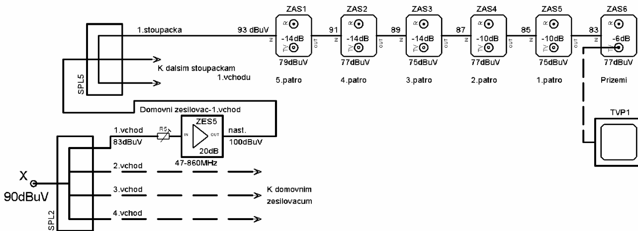
Obr. 12. Domovní rozvod STA se stoupacím vedením
