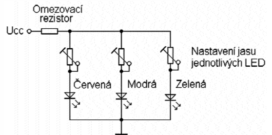
Obr. 4. Zdroj světla s nastavitelnou barvou
